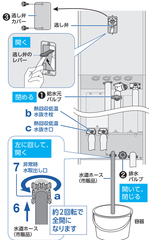
貯湯ユニット(配管カバーを取り外した状態) (イラストはすべての栓、バルブが「閉」の状態を表示)
