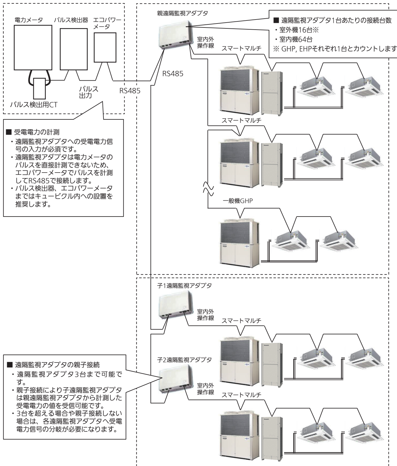
図1 スマートマルチの基本的なシステム構成
