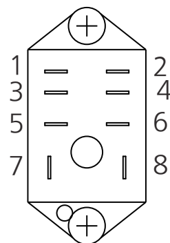
補助リレー端子配置図
