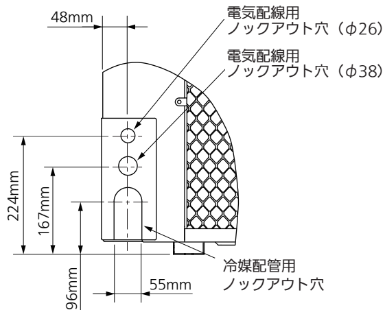
A矢視(冷凍機背面 配管・配線用穴)
