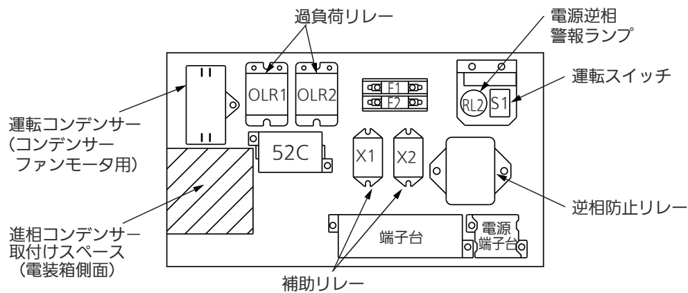
電装箱内部部品配置図
