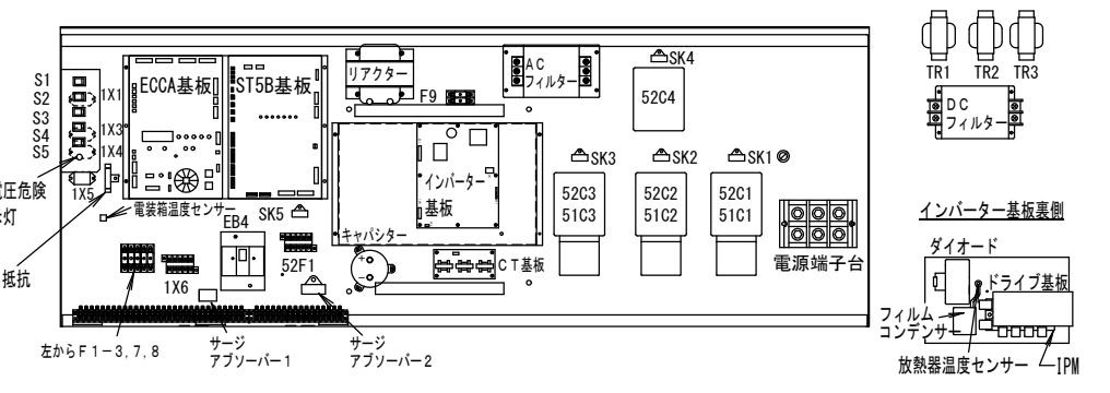
電装箱内部品配置図
