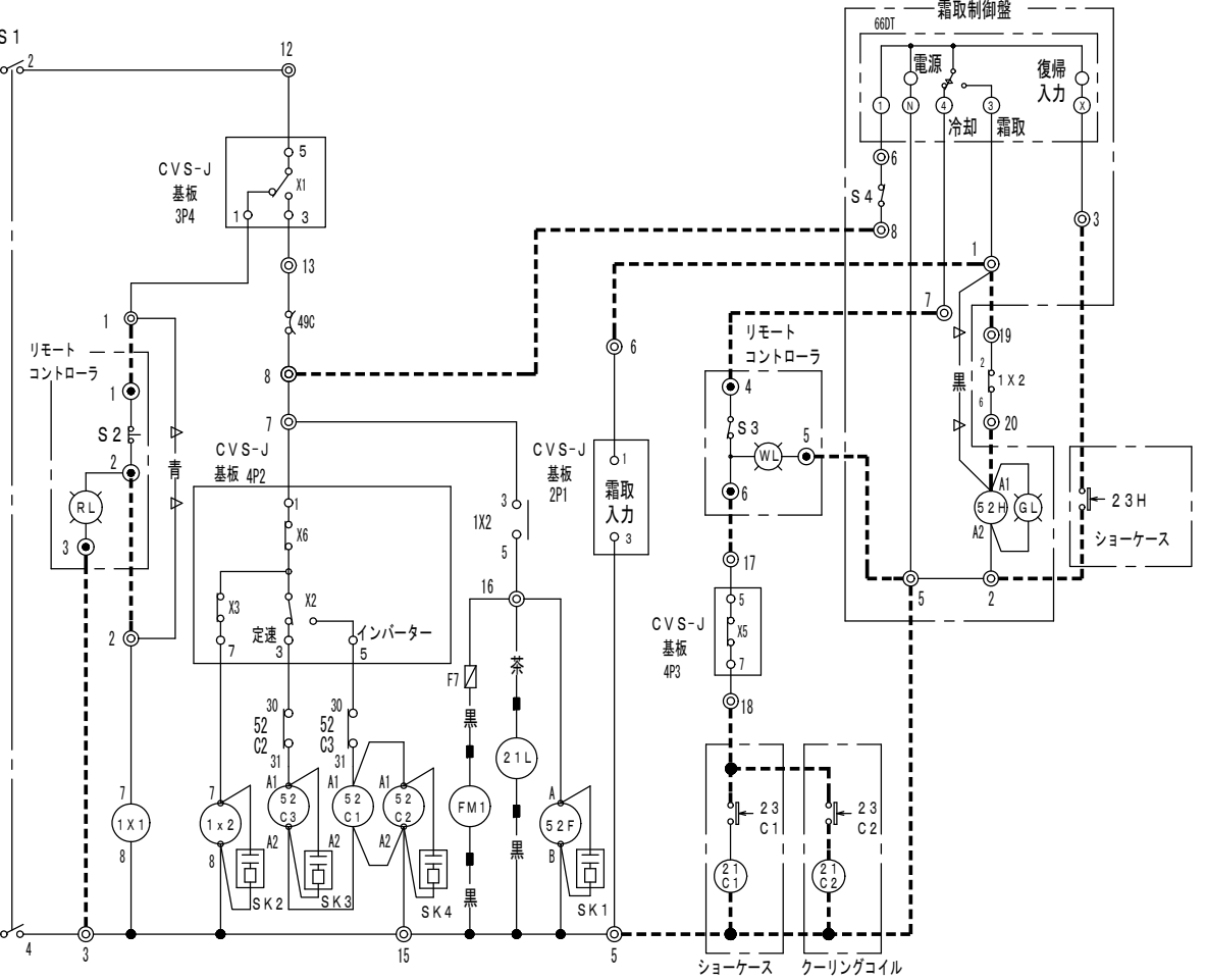
<霜取制御盤SDT-601Mを使用する場合の回路例>
