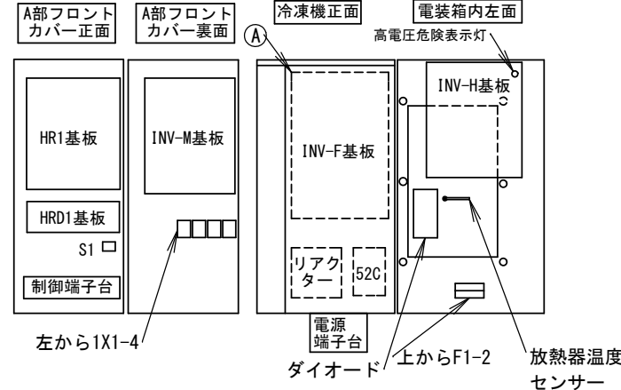
電装箱内部部品配置図
