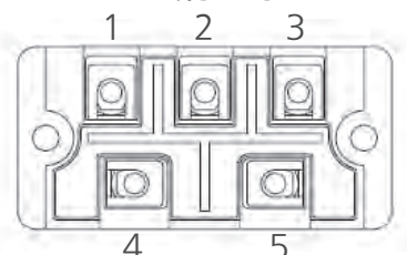
ダイオード端子配列
