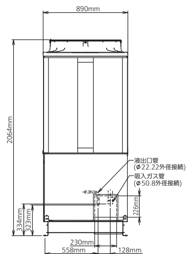
冷凍機右側面
