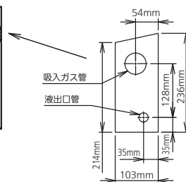
冷凍機下面配管用穴 詳細
