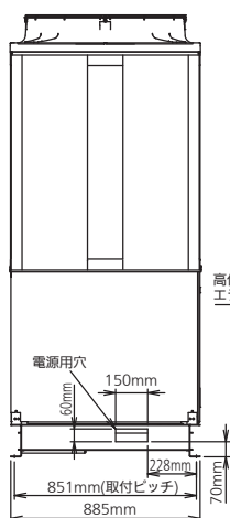
冷凍機左側面
