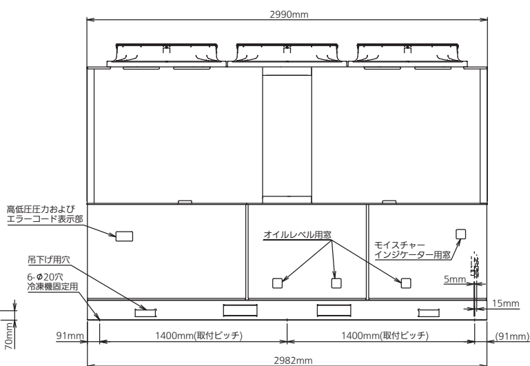
冷凍機正面
