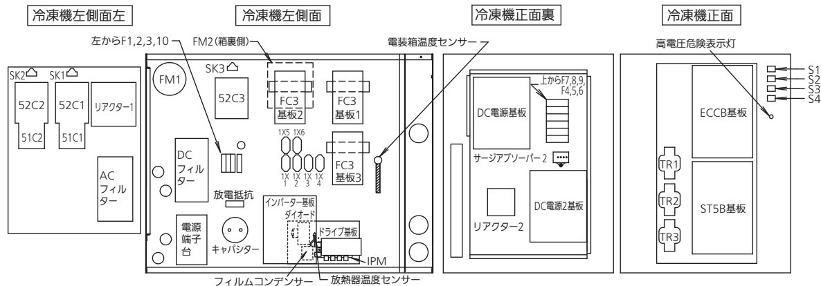
電装箱内部部品配置図
