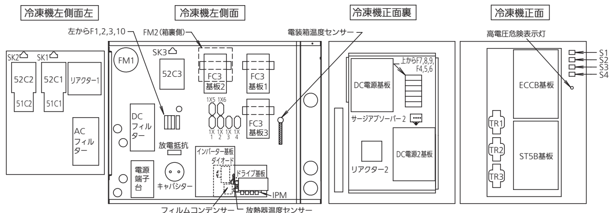
インバーター部の電気部品配置図
