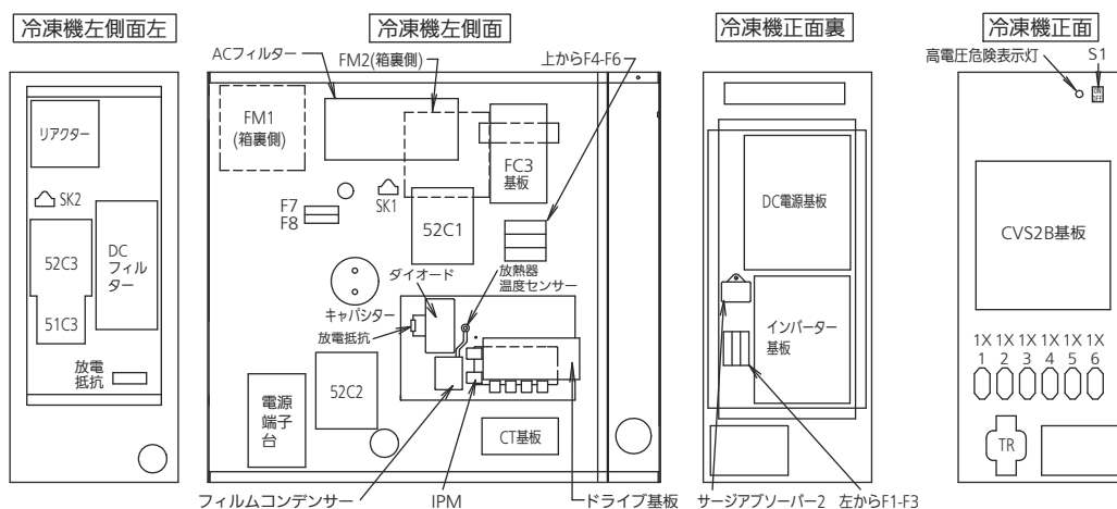
電装箱内部部品配置図
