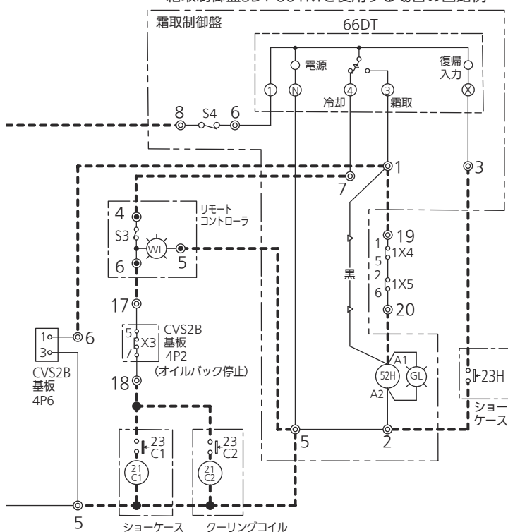
<霜取制御盤SDT-601Mを使用する場合の回路例>
