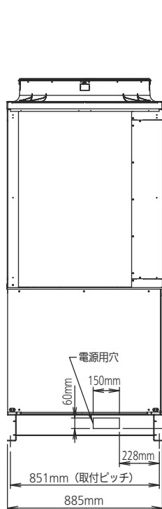
冷凍機左側面
