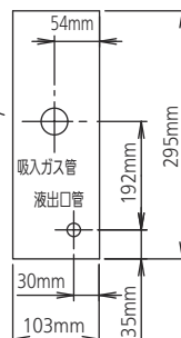
冷凍機下面配管用穴 詳細
