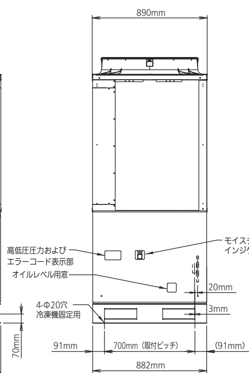
冷凍機正面
