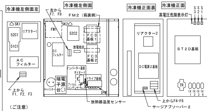
電装箱内部部品配置図
