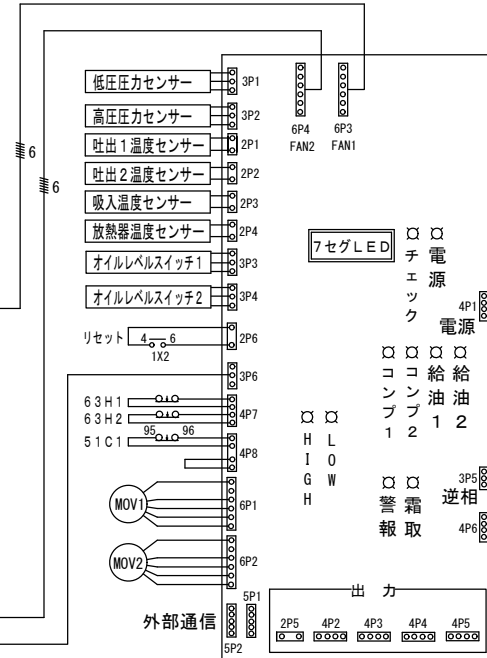
ST2D基板入出力端子
