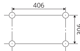
取り付け寸法(単位 mm)
