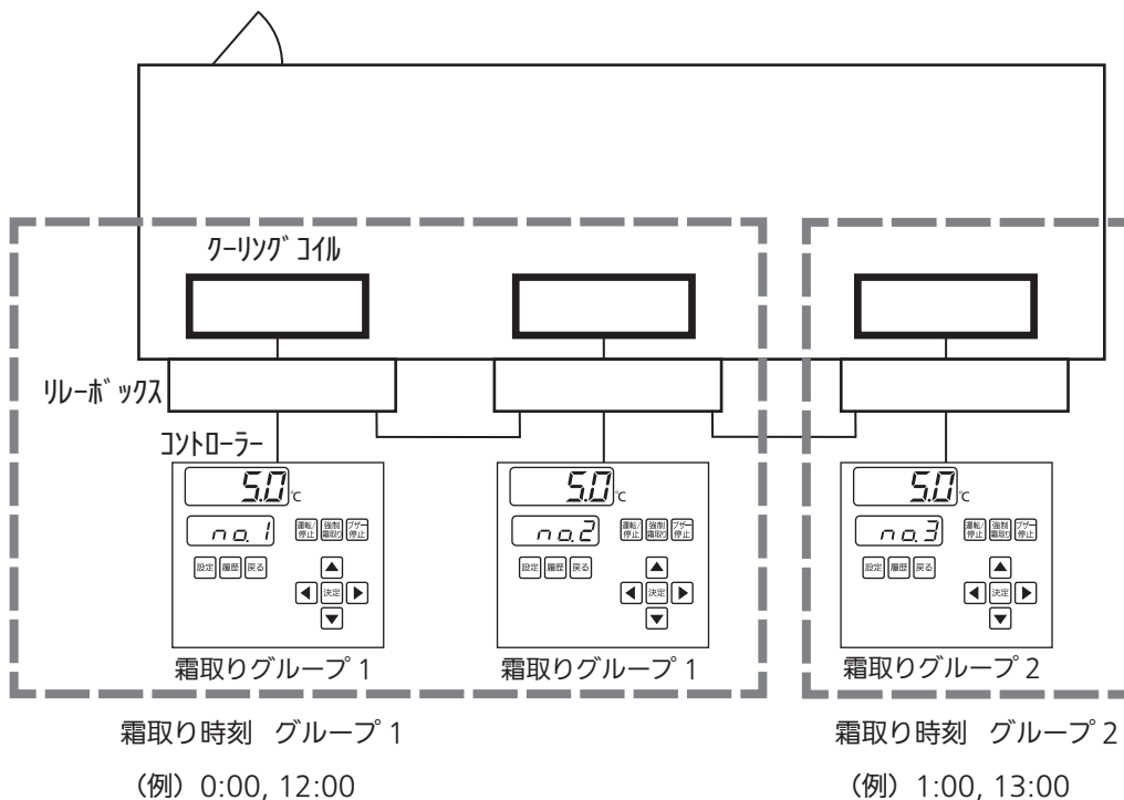
リレーボックスNo1,2で霜取り同期する場合
