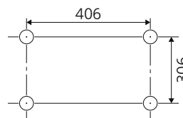
取り付け寸法(単位 mm)
